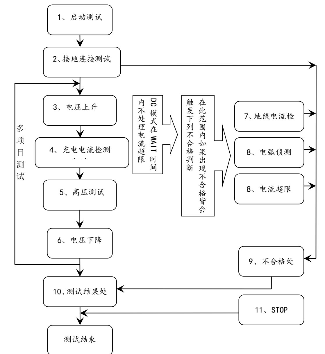
图 4-1 仪器的测试流程
