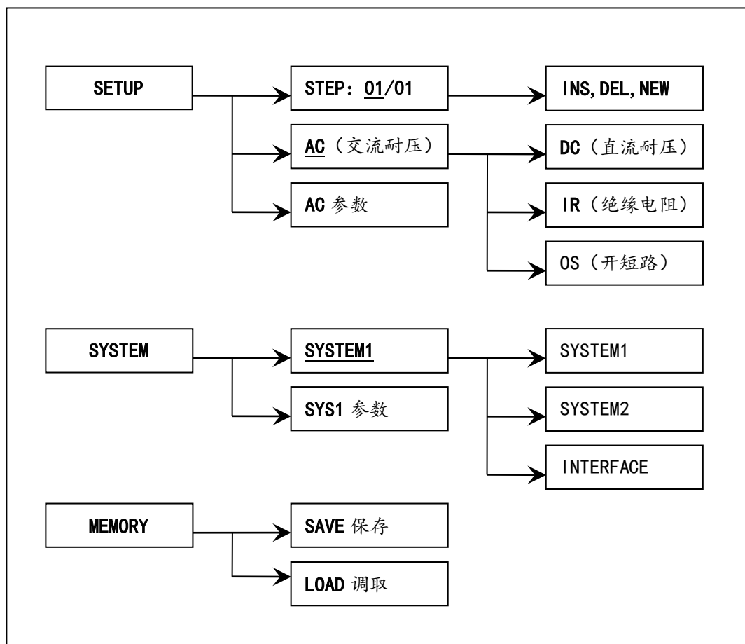
图 3-1 测试操作流程示意图
