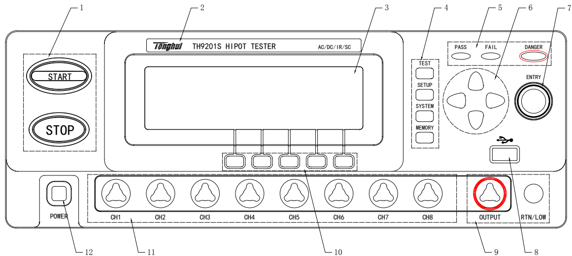
图 2-1 前面板样式
