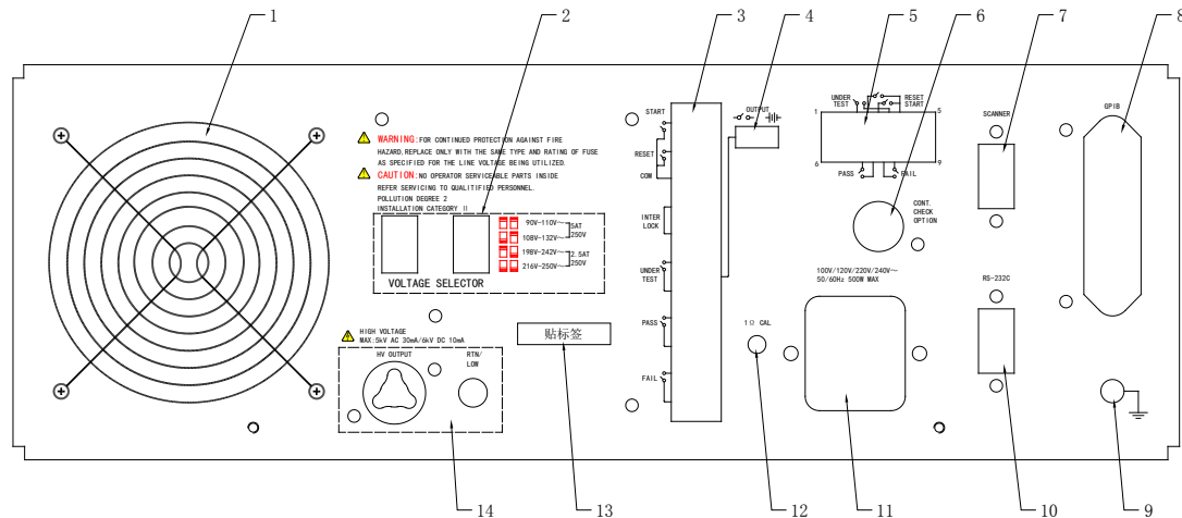
图 2-2 后面板样式
