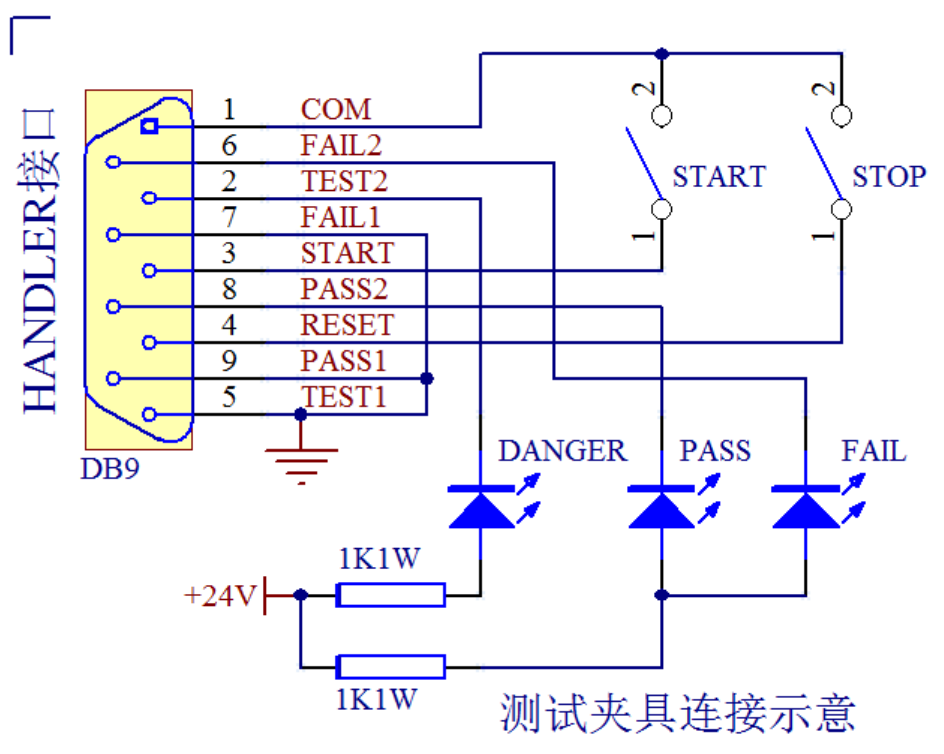
图 4-4 HANDLER 外部电路连接示意图（外接电源）
