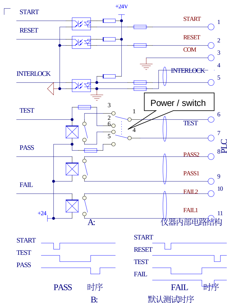
4-2 PLC 接口结构与时序
