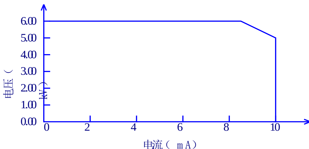
图 2-4 TH9201/S 直流电压输出范围
